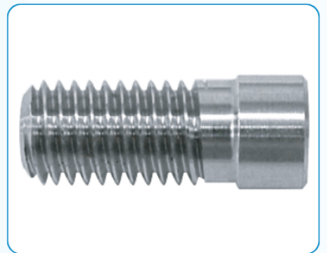
材質:SUS304 特殊六角穴付小頭ボルト 1/4-28UNFX1/2 2条ねじ
