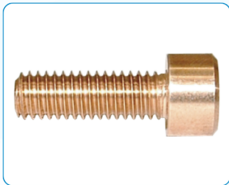
材質:リン青銅 六角穴付ボルト M6X18 φ2.0貫通穴
